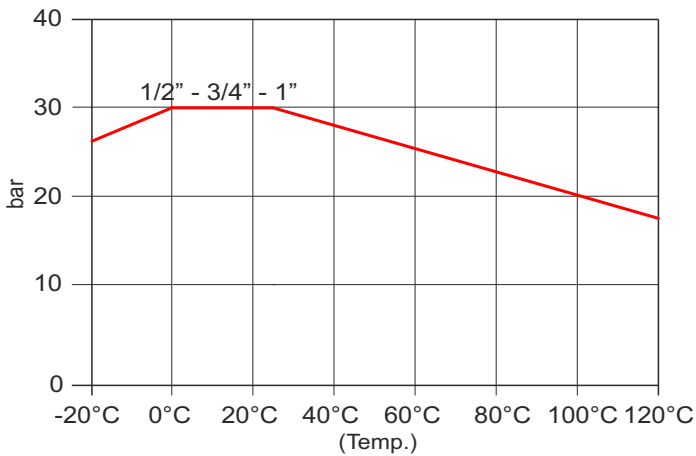
Diagramma pressione / temperatura Diagrama presiune/temperatura
