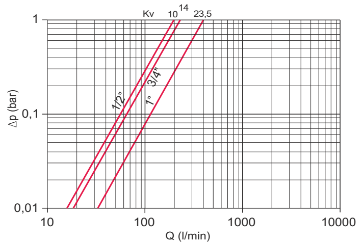
Diagramma portata/perdita di carico Diagrama fluxului/pierderii de sarcina
