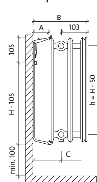
tip FHV 30
