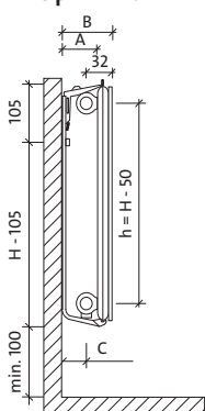
tip FHV 10
