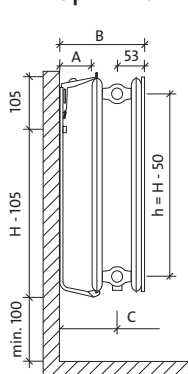
tip FHV 20
