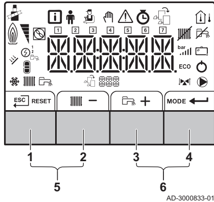
Fig.1 Tablou de comandă
