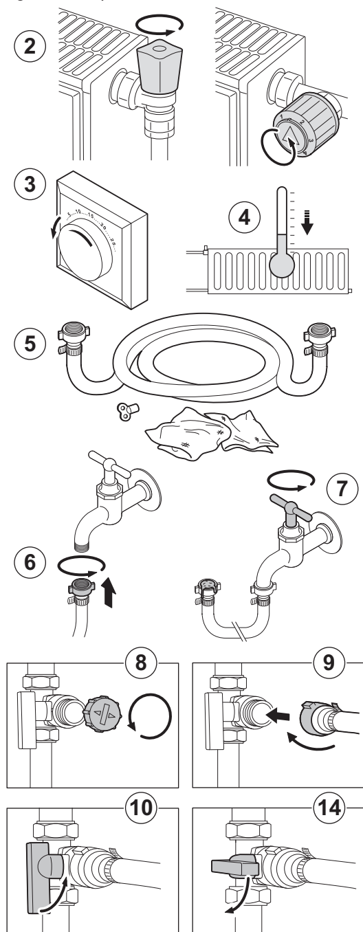
Fig.35 Umplerea sistemului
