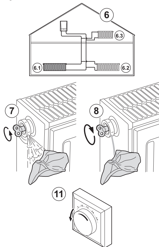
Fig.38 Aerisirea sistemului
