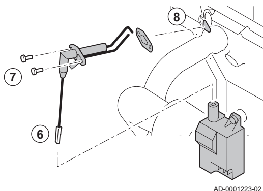
Fig.132 Înlocuirea electrodului de ionizare/aprindere
