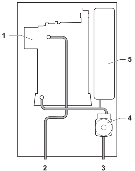
Fig.3 Calenta Ace 15S - 25S
