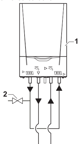
Fig.12 Utilizarea ca boiler
