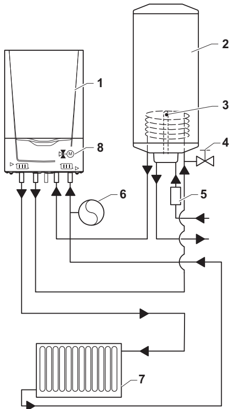
Fig.11 Conectarea boilerului cu o vană cu trei căi
