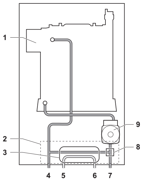
Fig.8 Calenta Ace 40C
