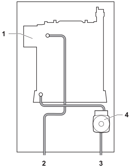
Fig.4 Calenta Ace 35S
