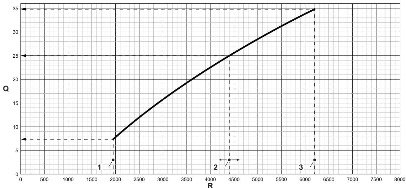
Fig.123 Grafic pentru Calenta Ace 35S - 35DS - 40C
