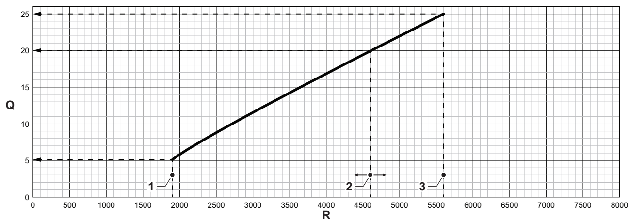
Fig.122 Grafic pentru Calenta Ace 25S - 25DS - 28C
