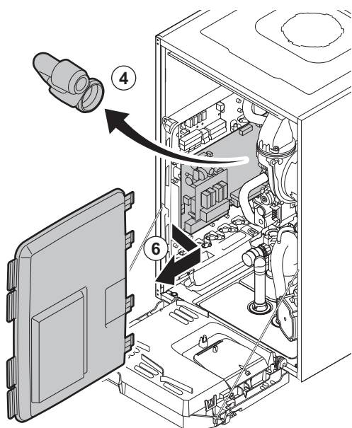
Fig.155 Acces la plăcile electronice
