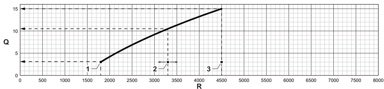
Fig.121 Grafic pentru Calenta Ace 15S - 15DS
