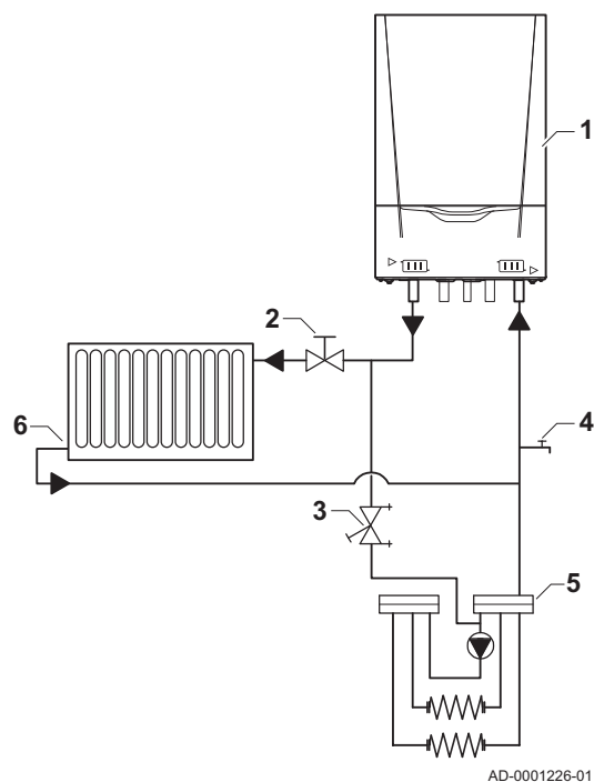
Fig.9 Racordarea încălzirii prin pardoseală
