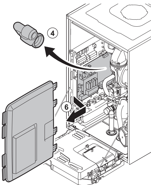
Fig.23 Acces la placa electronică.
