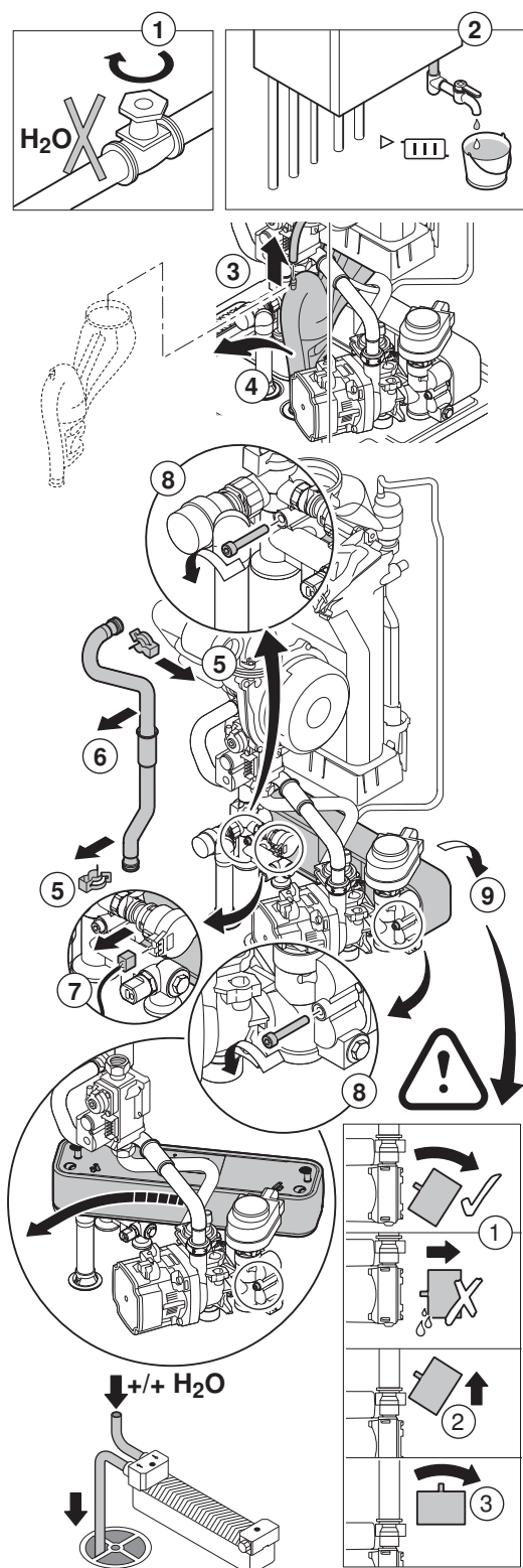
Fig.133 Curățarea schimbătorului de căldură cu plăci
