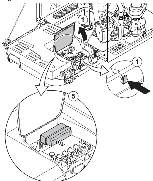
Fig.13 Accesul la conectori
