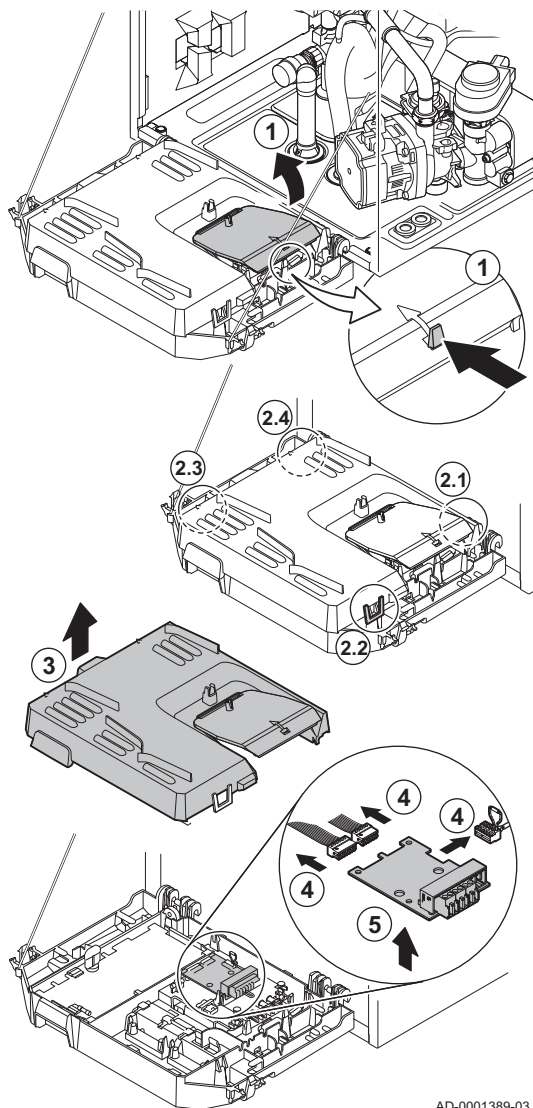
Fig.139 Accesul la conectori
