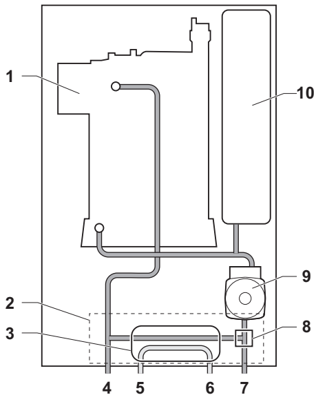
Fig.7 Calenta Ace 28C
